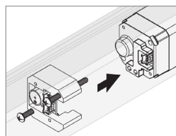
QEL-B Kit
